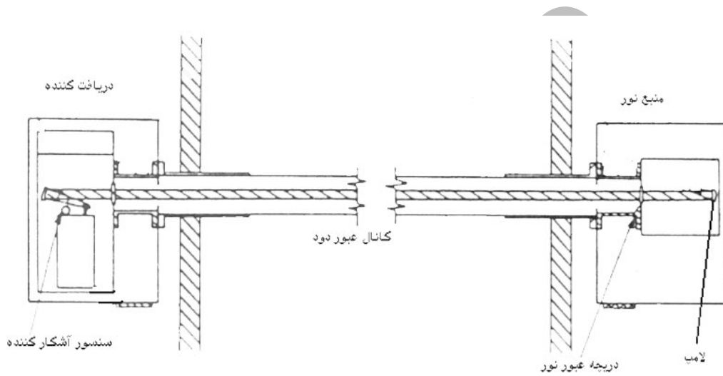
شکل ۱: طرحواره دستگاه سنجش دود
