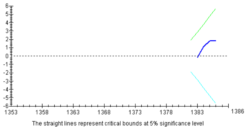
نمودار ۷- مجموع تجمعی پسماندهای برگشتی استاندارد شده تابع تقاضای پول (Cusum)
