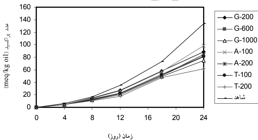
شکل شماره ۳- مقایسه تیمارهای عصاره متانولی بخش گوشت پایه سیترومولو با آنتی‌اکسیدان‌های سنتزی از نظر میزان عدد پراکسید
