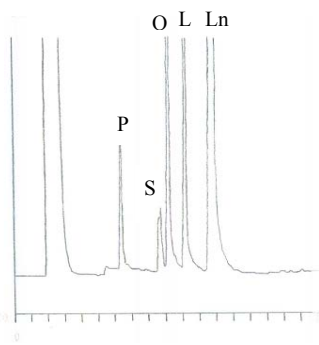
شکل شماره ۹- کروماتوگرام متیل استر اسیدهای چرب روغن بزرک در مرحله آخر جزء به جزء سازی با استفاده از دستگاه GC اسید لینولئیک: L اسید لینولئیک (Ln):
