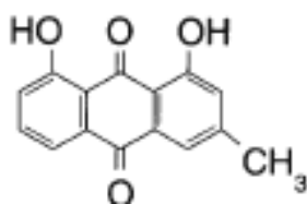
Chrysofanol
