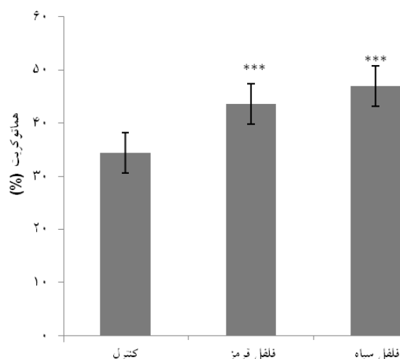
نمودار شماره ۴ - مقایسه مقدار هماتوکریت (درصد حجمی گلبول‌های قرمز)، در گروه‌های دریافت‌کننده فلفل قرمز و سیاه با گروه کنترل (n=7). هر ستون بیانگر میانگین ± متوسط انحراف از معیار (Mean ± SEM) است. تفاوت معنی‌دار گروه‌های دریافت‌کننده فلفل قرمز و دریافت‌کننده فلفل سیاه با کنترل (p < 0/01) نشان داده شده است. (**=)
