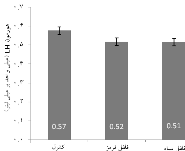
نمودار شماره ۲- میزان هورمون LH در گروه‌های تیمار با فلفل قرمز و سیاه در مقایسه با گروه کنترل (n=7). هر ستون بیانگر میانگین \pm متوسط انحراف از معیار (Mean \pm SEM) است. با وجود کاهش جزئی در گروه‌های تحت تیمار، تفاوت معنی‌دار نیست.
