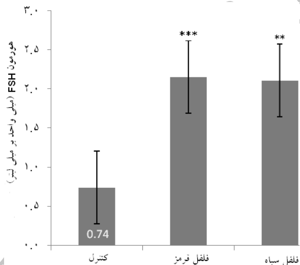
نمودار شماره ۳- مقایسه میزان هورمون FSH، در گروه‌های دریافت‌کننده فلفل قرمز و سیاه با گروه کنترل (n=7). هر ستون بیانگر میانگین \pm متوسط انحراف از معیار (Mean \pm SEM) است. تفاوت معنی‌دار گروه دریافت‌کننده فلفل قرمز با گروه کنترل ( p < 0.001 ) و گروه دریافت فلفل سیاه با کنترل ( p < 0.01 ) نشان داده شده است.
