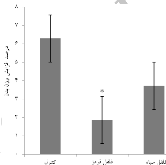
نمودار شماره ۵ - مقایسه اثر فلفل قرمز و سیاه بر میزان افزایش وزن بدن، (n=7). هر ستون بیانگر میانگین ± متوسط انحراف از معیار (Mean ± SEM) است. تفاوت معنی‌دار گروه دریافت‌کننده فلفل قرمز با گروه کنترل (p < 0/05) نشان داده شده است. (*=)
