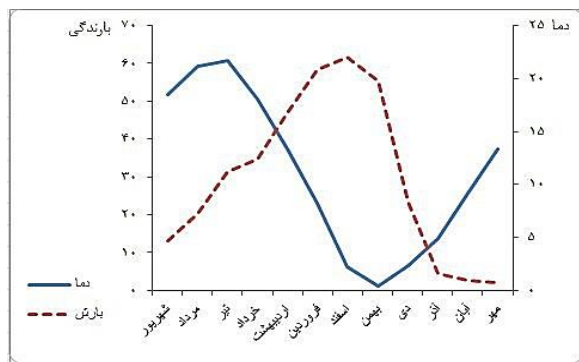
شکل شماره ۲- منحنی آمیروترمیک منطقه مورد مطالعه
