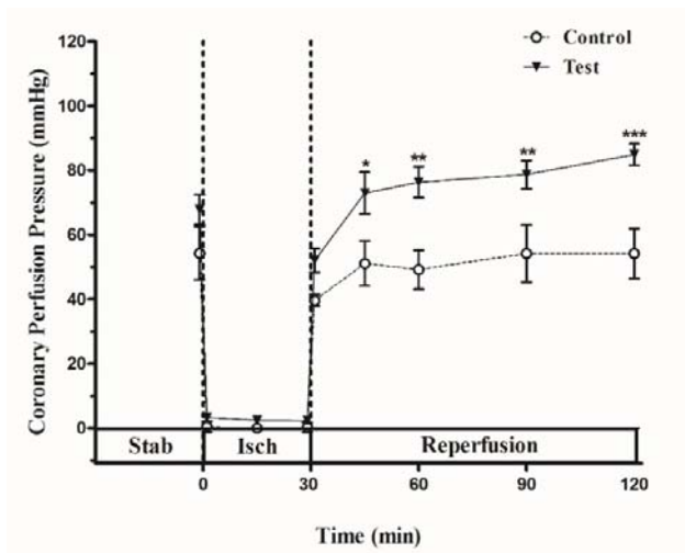
نمودار شماره ۵- تأثیر عصاره پیه انار بر فشار پرفوزیون قلب ایزوله. عصاره پیه انار و دارونما به مدت ۳ هفته به ترتیب به رت‌های آزمون و شاهد گاوآژ شد. سپس قلب ایزوله رت‌ها تحت شرایط ایسکمی (۳۰ دقیقه) و پرفوزیون مجدد (۹۰ دقیقه) مورد مطالعه قرار گرفت (n=۱۰). علامت ستاره بیانگر اختلاف معنی‌دار (*): P < 0/05 , **: P < 0/01 و ***: P < 0/001 بین دو گروه می‌باشد.
