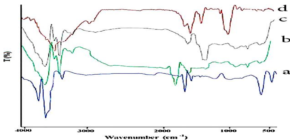
شکل ۳. نمودار طیف‌سنجی مادون قرمز با تبدیل فوریه فیلم‌های با و بدون عصاره هیدروالکلی گیاه کک کش بیابانی کیتوزان-ژئین
