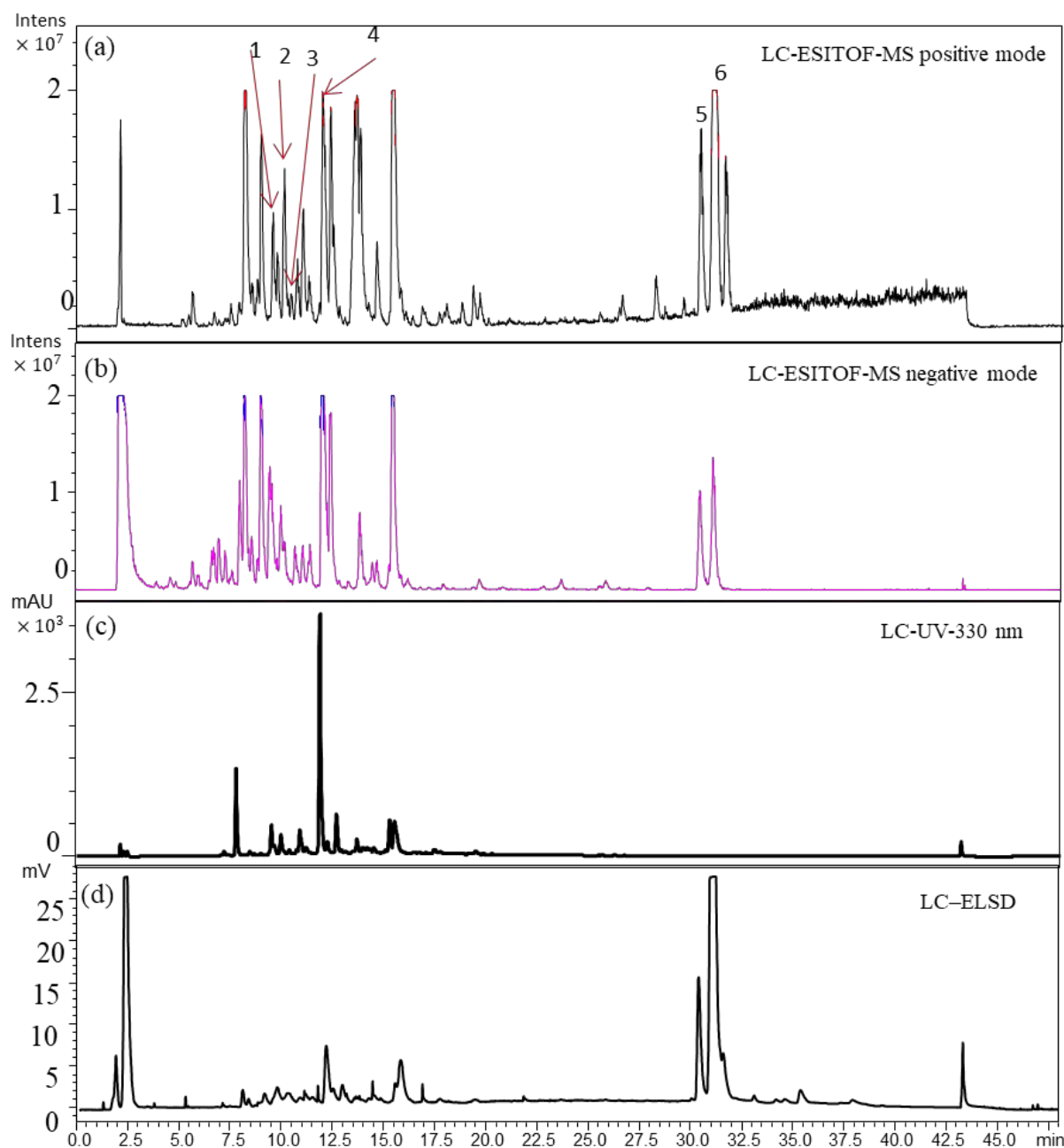
شکل ۷. طیف HPLC-UV-MASS-ELSD عصاره متانولی گیاه آویشن شیرازی و ترکیبات شناسایی شده که در طیف MASS شماره گذاری شده‌اند.
