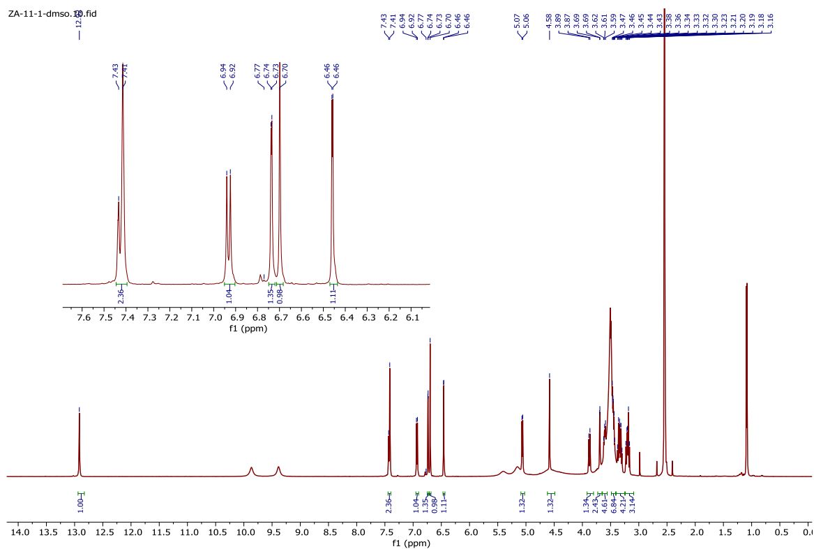
شکل ۲. طیف ^1H NMR ترکیب شماره ۱، Luteolin 7-O-rutinoside (طیف سنج ۵۰۰ مگا هرتز، حلال DMSO دو تهره)
