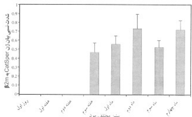
شماره ۱: شدت نسبی محصول RT-PCR برای ژن CatSper بر سنین مختلف موش. اندازه‌گیری در هر گروه سنی به صورت نسبت شدت باند CatSper به باند \beta 2m می‌باشد و نتایج به صورت Mean \pm SE نشان داده شده است.
