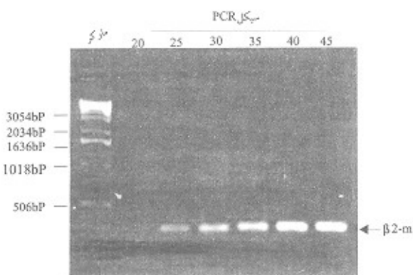
شکل ۳. طرح الکتروفورزی محصول RT-PCR مربوط به انتخاب تعداد سیکل PCR روی ژن \beta 2m (ستون ۱، مارکر و ستونهای ۲ تا ۵، به ترتیب محصول سیکلهای ۲۰، ۲۵، ۳۰، ۳۵، ۴۰، ۴۵ را نشان می‌دهد)
