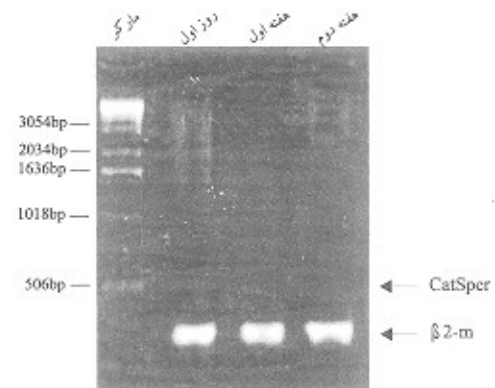
شکل ۴: طرح الکتروفورزی محصول RT-PCR با تعداد سیکل ۴۵ برای ژنهای \beta 2m و CatSper ستون ۱ تا ۳ به ترتیب مربوط به گروه سنی یک، دو و سه تا دو هفته می‌باشد.
