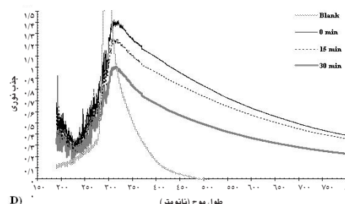
شکل ۳: اثر پلاسمای تولید شده توسط الکتروود تخت (A) و شانه‌ای (B) آلومینیومی با منبع تغذیه DC و الکتروود تخت (C) و شانه‌ای (D) آلومینیومی با منبع تغذیه AC بر باکتری E. coli در زمان‌های متفاوت
