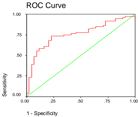
نمودار ۱- ROC Curve مساسیت و اختصاصیت NAG ادرار در تشفیص پیلونفریت ماد
