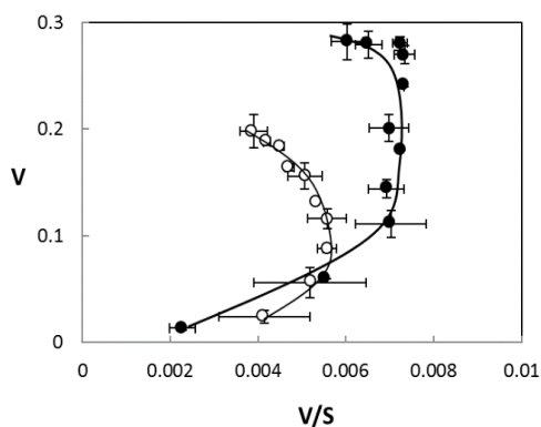
شکل ۴: منحنی هیل برای آنزیم آدنوزین دآمیناز بدون کافئین (دایره توپر) و به همراه کافئین 10mM (دایره توخالی). با استفاده از شیب نمودار هیل (ضریب هیل) و طول از مبدا آن ( S_{1/2} ) مقدار اثر آلوستریک مثبت اندازه گیری و ارزیابی شد. نتیجه این اندازه گیری ها در جدول ۱ خلاصه شده است.
