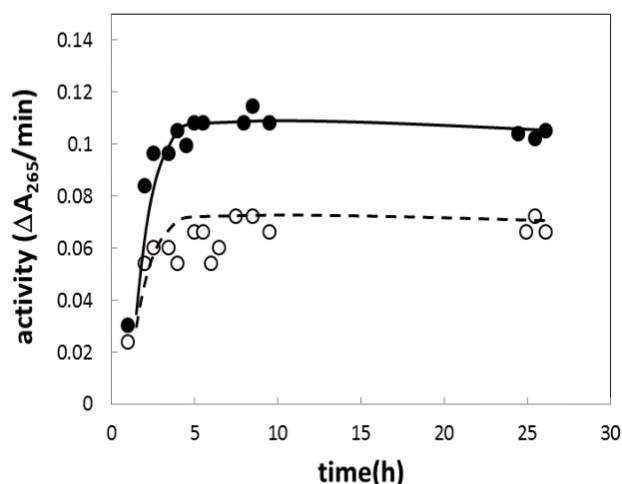
شکل ۵: تغییرات V_{max} آنزیم آدنوزین دآمیناز به عنوان تابعی از زمان انکوباسیون، بدون کافئین (دایره توپر) و به همراه کافئین 10 mM (دایره تو خالی).
