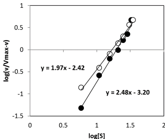
شکل ۳: منحنی ادی-هافستی آدنوزین دآمیناز بدون کافئین (دایره توپر) و به همراه کافئین 10mM (دایره توخالی). با توجه به شکل ۳، وجود کافئین شدت اثر آلوستریک مثبت را تغییر داده است. برای کمی کردن شدت اثر آلوستریک
