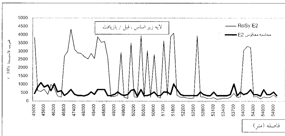
شکل ۶ مقایسه ضرایب ارتجاعی حاصل از محاسبه معکوس و نتایج RoSy برای قشر اساس، قبل از بازافت (با رویه)
