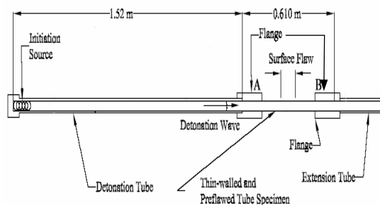
شکل ۳ لوله انفجار [۱]
