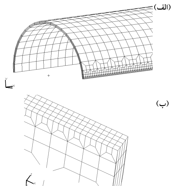
شکل ۷- (الف) هندسه مش‌بندی برای مدل‌سازی لوله ترک‌دار
