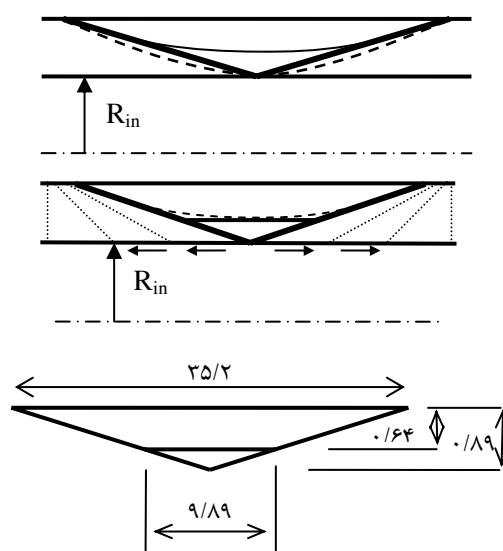
شکل ۲۰ ترک نیم بیضوی رشد یافته که به صورت ترک راه بدر مثلثی شکل در نظر گرفته شده است (اندازه ها به میلی متر)
