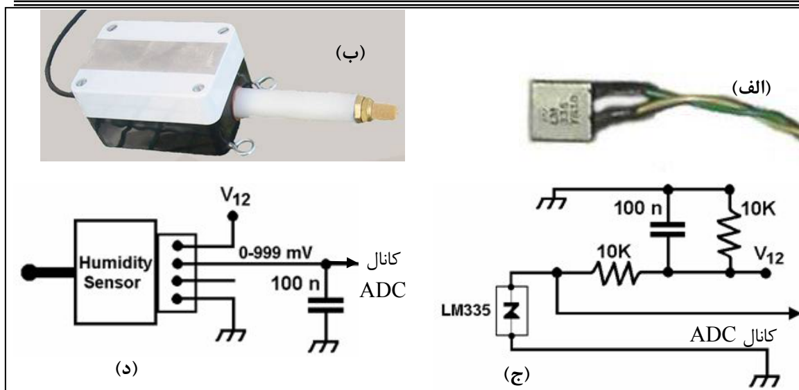
شکل شماره ۷- سنسورهای استفاده شده. (الف) سنسور دما LM335 و (ب) سنسور رطوبت نوع خازنی، (ج) مدار واسط اتصال سنسورهای دما به میکروکنترلر و (د) مدار واسط اتصال سنسور رطوبت به میکروکنترلر
