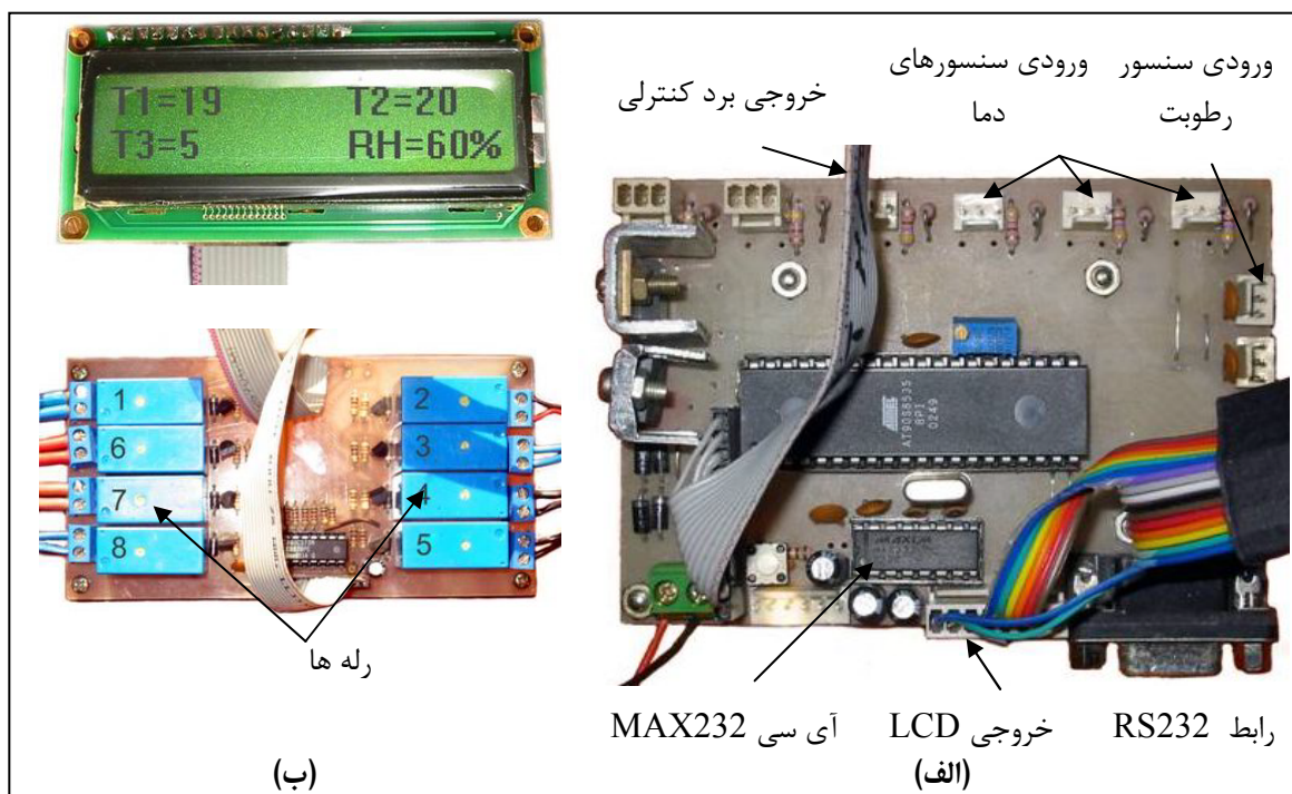
شکل شماره ۵- میکروکنترلر (الف) برد اصلی و (ب) نمایشگر LCD (بالا) و برد کنترل (پایین)
