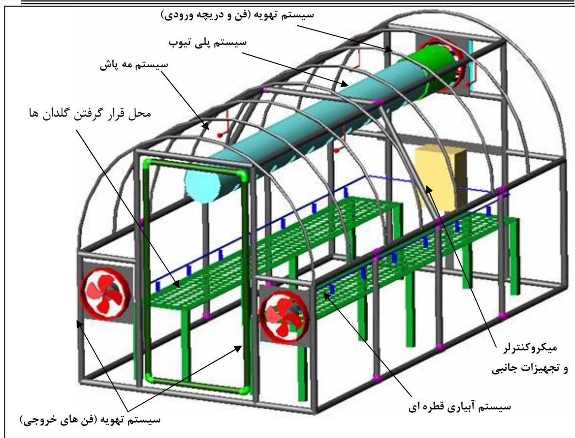
شکل شماره ۲- نمایی از گلخانه مدل طراحی شده و تجهیزات کنترلی آن
