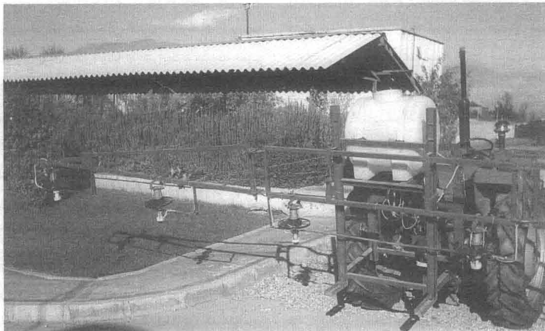
شکل شماره ۲- سمپاش بوم دار تراکتوری مجهز به صفحات چرخان
