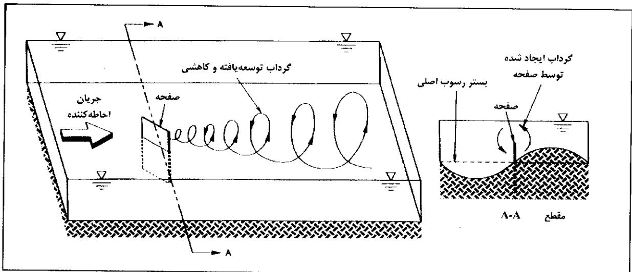
شکل شماره ۲- شیوار آب شستگی ایجاد شده بر اثر صفحه مستغرق جلو دهانه آبیگر (Barkdoll, 1997)
