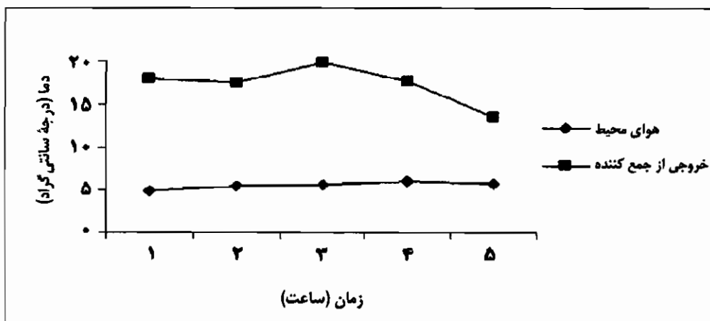
شکل شماره ۶- مقایسه دمای هوای محیط و هوای خروجی از جمع‌کننده در تاریخ ۱۳۸۳/۹/۴
