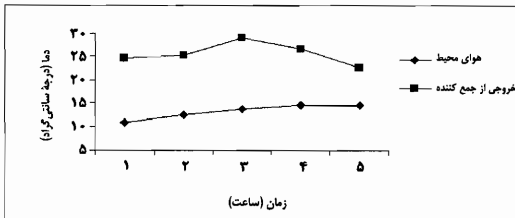
شکل شماره ۴- مقایسه دمای هوای محیط و هوای خروجی از جمع‌کننده در تاریخ ۱۳۸۲/۸/۳۰
