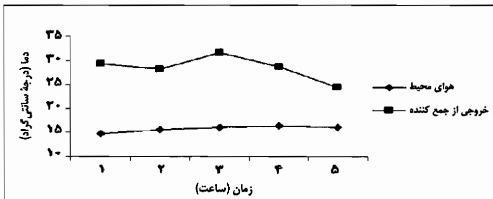
شکل شماره ۵- مقایسه دمای هوای محیط و هوای خروجی از جمع‌کننده در تاریخ ۱۳۸۳/۹/۲
