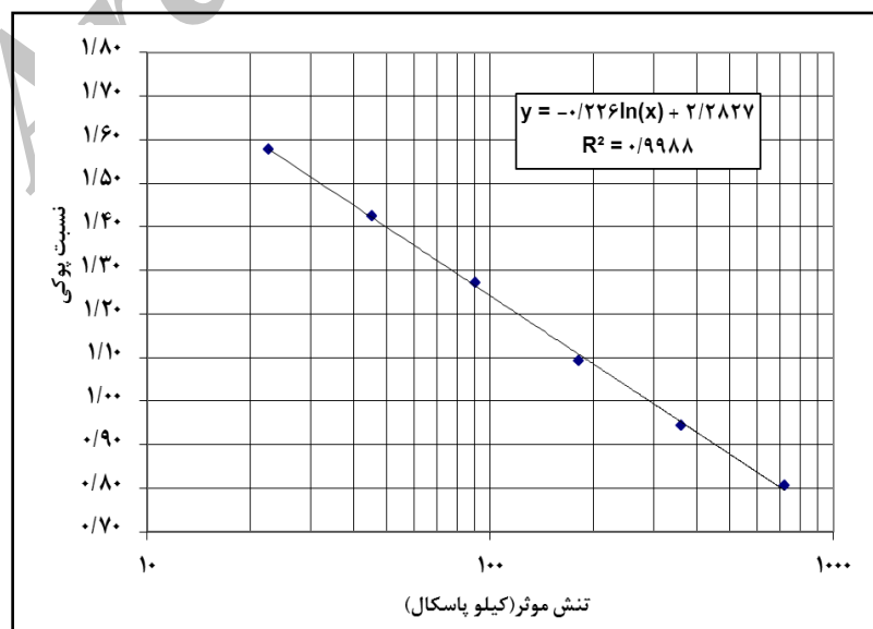
شکل ۴- منحنی تنش مؤثر - نسبت پوکی برای نمونه حاوی ۱ درصد کربنات سدیم
