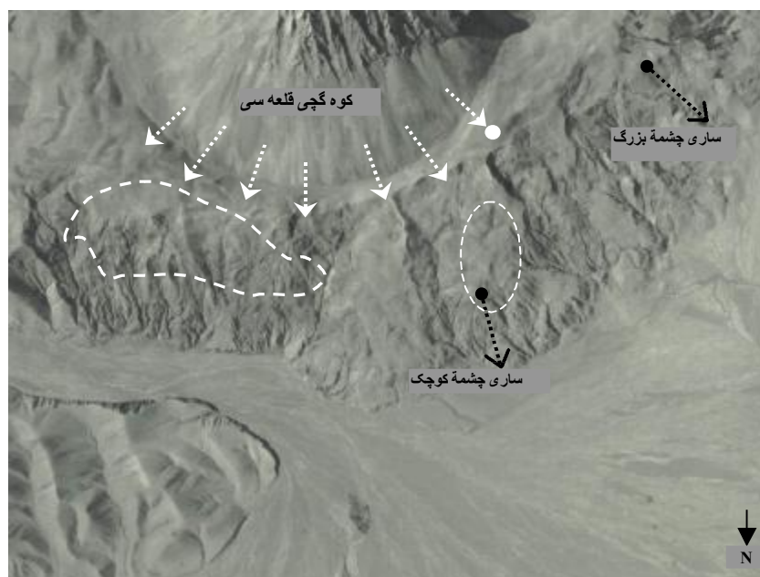
شکل ۶ مورفولوژی عناصر برجای گذاشته شده در روی زبانه یکی از لغزشها (داخل بیضی)، که در داخل یک زخمه لغزشی بزرگ واقع شده است.
