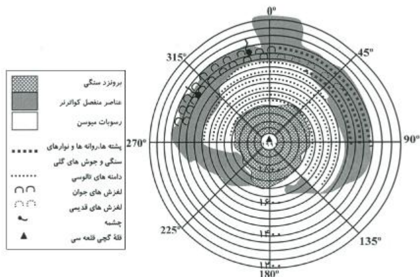
شکل ۲ موقعیت ارتفاعی پدیده‌های ژئومورفولوژیکی پریگلاسیری در مجاورت کوه گچی قلعه سی با تأکید بر جهت دامنه‌ها
