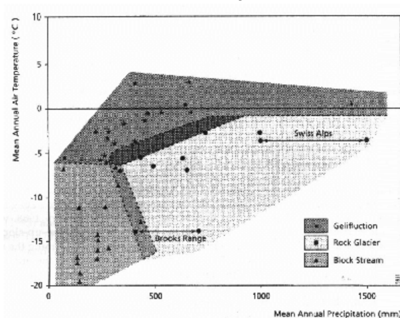
شکل ۷ رابطه بین آب و هوا و چشم‌اندازهای آلبی از نظر پراکندگی اشکال پریگلاسیری مثل روانه‌های سنگی فعال، یخچالهای سنگی فعال و سولیفلوکسیون/ ژلیفلوکسیون (هریس، ۱۹۹۴)
