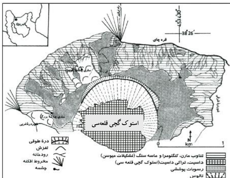
شکل ۱ نقشه زمین‌شناسی و ژئومورفولوژی منطقه مورد مطالعه
