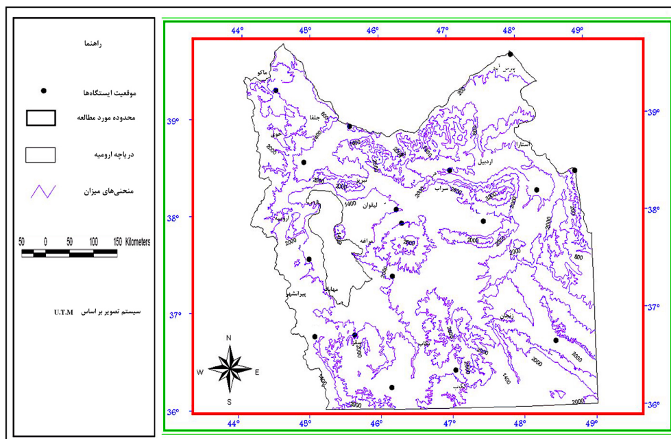
شکل ۱ نقشه توپوگرافی شمال غرب کشور به همراه موقعیت ایستگاه‌های هواشناسی
