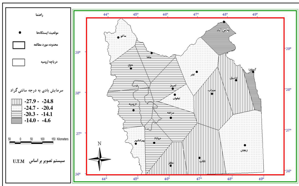
شکل ۸ ناحیه بندی از مقادیر حداقل مطلق سرماییش بادی در شمال غرب کشور به روش تیسسن
