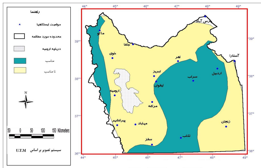
شکل ۱۱ انطباق لایه‌های سرمایش بادی و توپوگرافی در شمال غرب ایران
