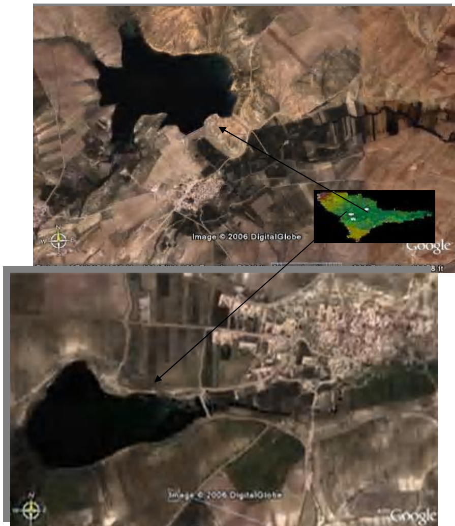
شکل 9: سدهای احداث شده درحوضه قرنقوچای واحتمال آسیب پذیری روستاهای پایین دست سدها به هنگام تخلیه ناگهانی آب پشت آنها ( www.earthgoogle.com )
