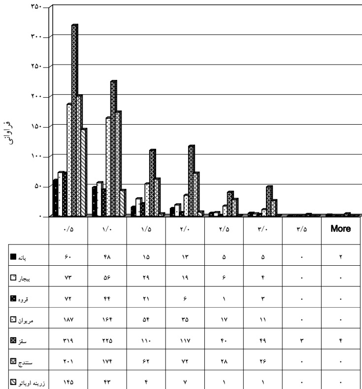
شکل ۱: فرآوانی ریزش برف غیر رگباری در دماهای بیش از صفر درجه سلسیوس، در ایستگاه‌های استان کردستان، طی دوره آماری موجود.
