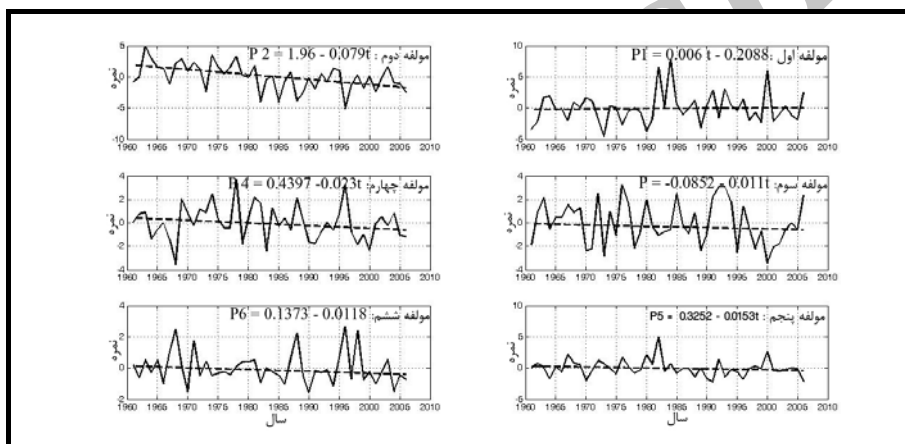
شکل ۱: تغییرات زمانی و روند شش مؤلفه مبنای نمایه‌های فرین بارش زنگان برای دوره آماری ۱۹۶۱-۲۰۰۶ (مأخذ: نگارنده)
