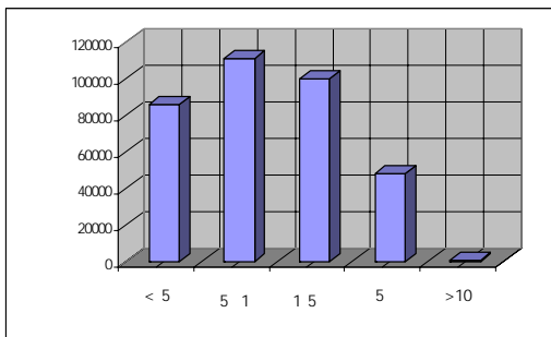
شکل ۱- نمودار هیستوگرام مربوط به نقشه وزنی نهایی زمین لغزش‌های حوضه سعیدآباد چای
