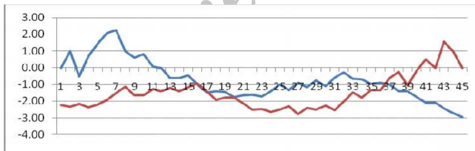
شکل ۱۲) نمودار \mu و \mu تاریخ خاتمه دمای صفر درجه سانتیگراد در ایستگاه یزد
