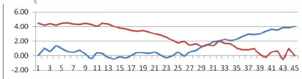
شکل ۶) نمودار u و t تاریخ آغاز دمای ۵ درجه سانتیگراد در ایستگاه یزد
