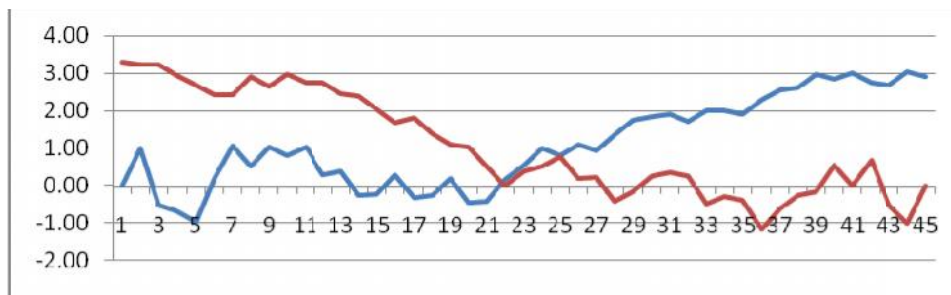
شکل ۱۰) نمودار \mu و \mu تاریخ آغاز دمای صفر درجه سانتیگراد در ایستگاه یزد
