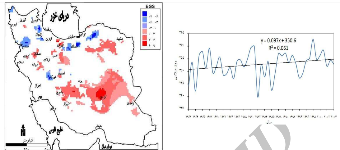
نگاره ۳) پراکنش مکانی مناطق دارای روند و شیب روند شاخص پایان دوره رشد (EGS) بر حسب مقدار در دهه (چپ) و روند شاخص برای کل ایران بر حسب مقدار در سال (راست)
