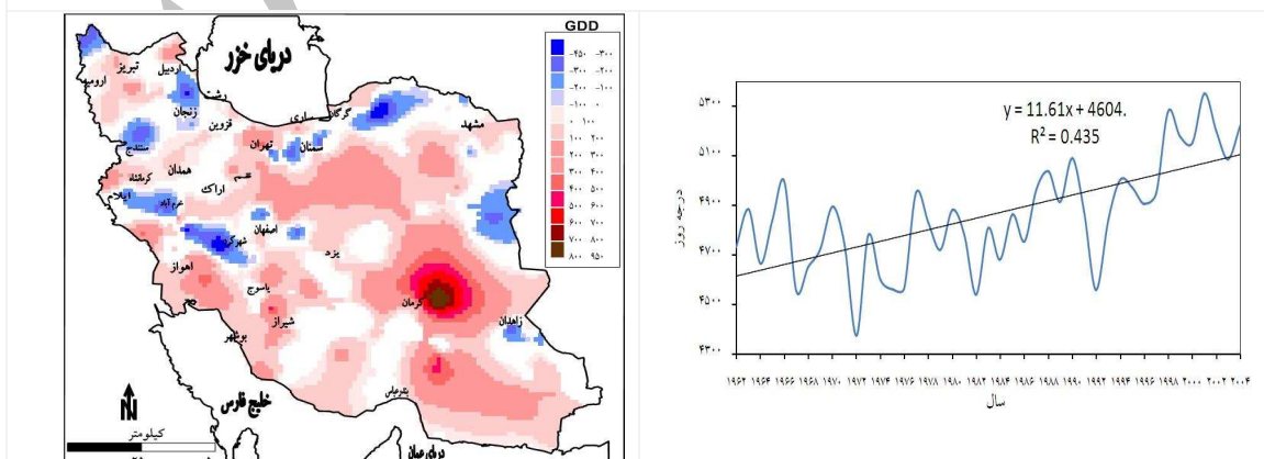
نگاره ۶) پراکنش مکانی مناطق دارای روند و شیب روند شاخص درجه روز رشد (GDD) بر حسب مقدار در دهه (چپ) و روند شاخص برای کل ایران بر حسب مقدار در سال (راست)
