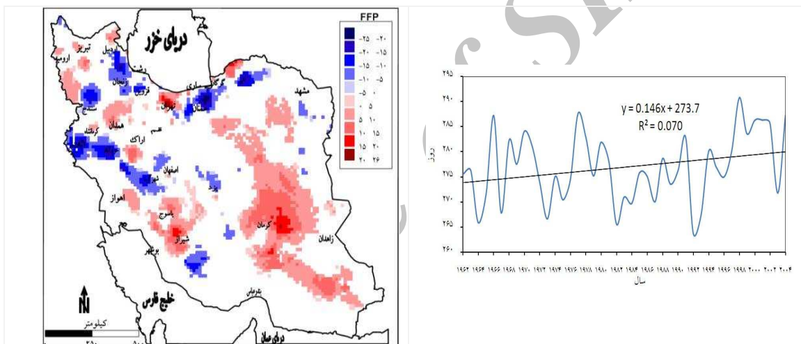
نگاره ۵) پراکنش مکانی مناطق دارای روند و شیب روند شاخص طول دوره یخبندان (FFP) بر حسب مقدار در دهه (چپ) و روند شاخص برای کل ایران بر حسب مقدار در سال (راست)
