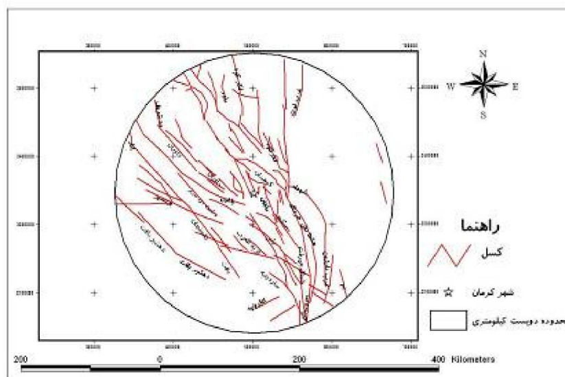
شکل (۲) گسل‌های محدوده ۲۰۰ کیلومتری شهر کرمان
