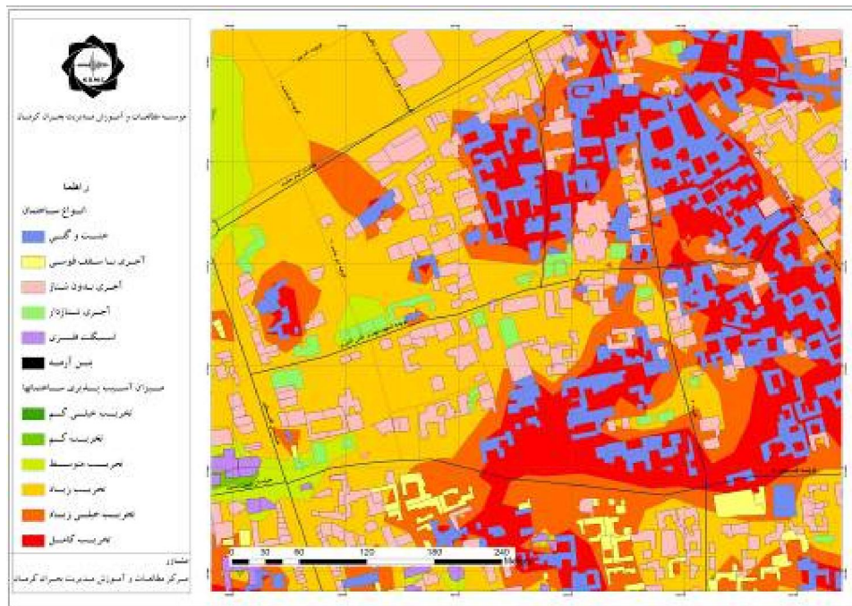
شکل ۹) نقشه آسیب پذیری سازه‌های و نوع سازه‌ها در ناحیه ۱۳
