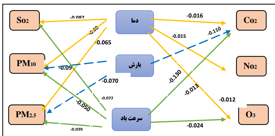
شکل ۲ - ضرایب بتای حاصل از تحلیل مسیر عوامل هواشناسی منتخب
