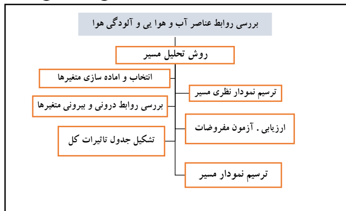
شکل ۴- روش کار در بررسی روابط تغییر آب‌وهوایی و آلودگی هوا
