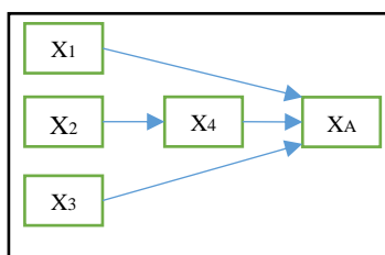
شکل ۳- نمونه نمودار مسیر با ۴ متغیر
