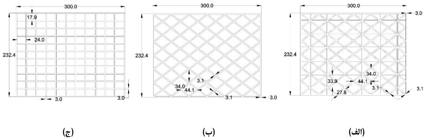
شکل ۲. هندسه هسته مشبک به همراه ابعاد الف) هسته مثلثی شکل ب) هسته لوزی شکل ج) هسته مربعی شکل. (کلیه ابعاد بر حسب میلیمتر است)
