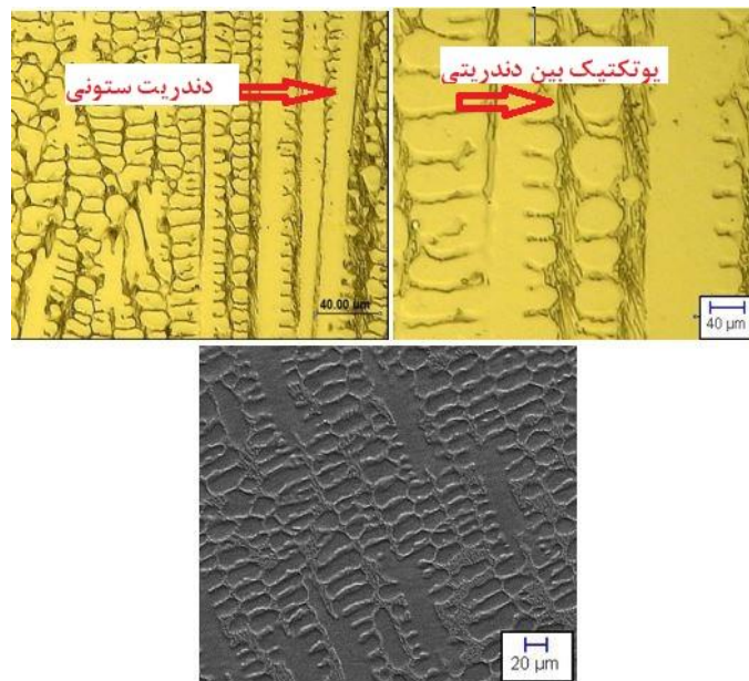
شکل ۱۰. تصاویر میکروسکوپی نوری و الکترونی لایه اول روکش کاری شده با استالیت ۶
