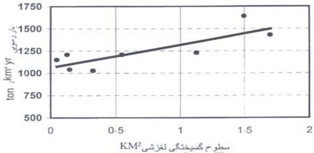
شکل-1- رابطه و همبستگی بار رسوبی و سطوح گسیختگی لغزشی در 8 زیر حوضه طالقان مرکزی
