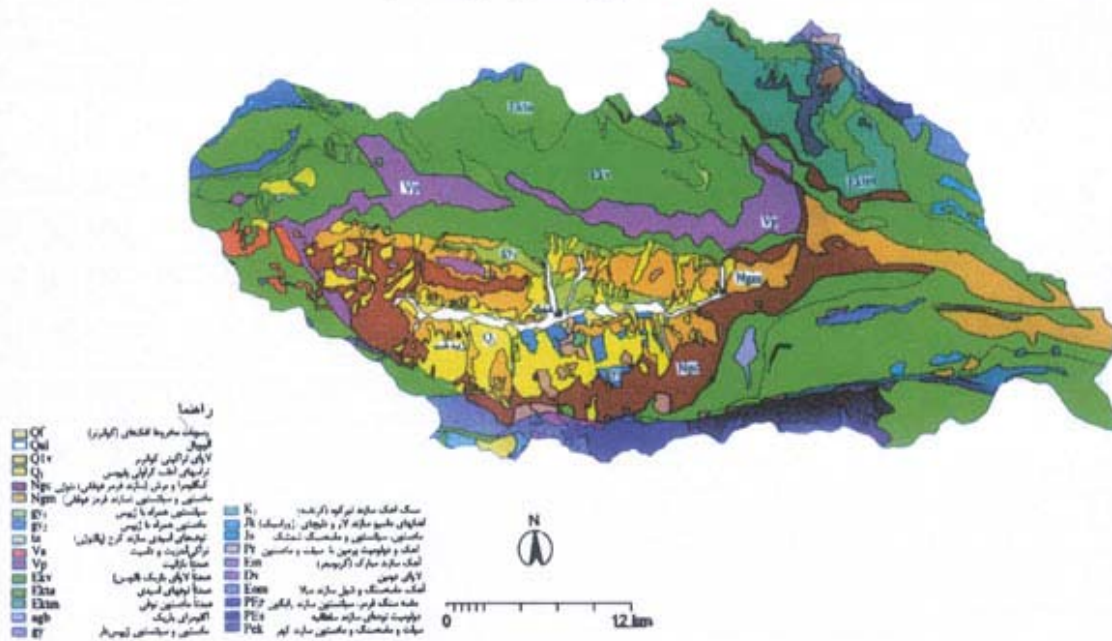
نقشه زمین شناسی حوزه طالقان
