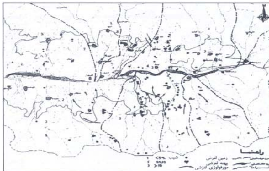
نقشه 2 - نقشه ثبت لغزش (Landslide Inventory Map) در حوضه طالقان مرکزی
