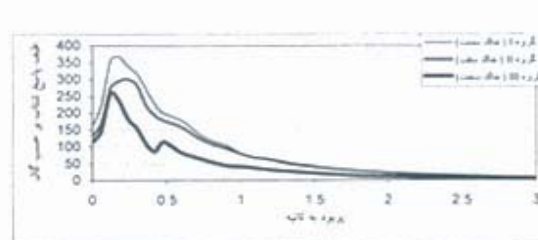
شکل 11- تغییرات طیف پاسخ شتاب قائم با پریود برای بزرگی 6/5 و فاصله رومگزی 10 کیلومتر
