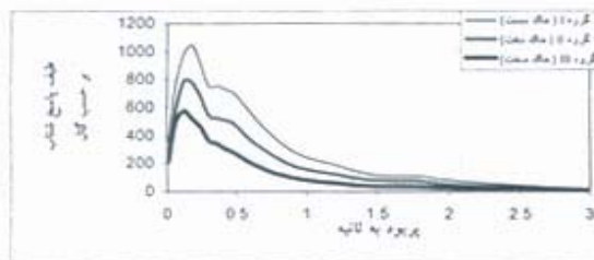
شکل 9- طیف پاسخ شتاب افقی برای بزرگی 6/5 و فاصله رومگزی 10 کیلومتر
