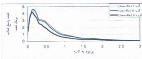
شکل 10- طیف پاسخ شمال شتاب افقی برای بزرگی 7 و فاصله رومگزی 10 کیلومتر
