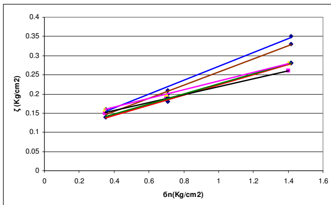
شکل ۱۰- نمودار مور-کولمب آزمایشهای برش مستقیم Cu انجام شده بر روی نمونه‌های بازسازی شده
