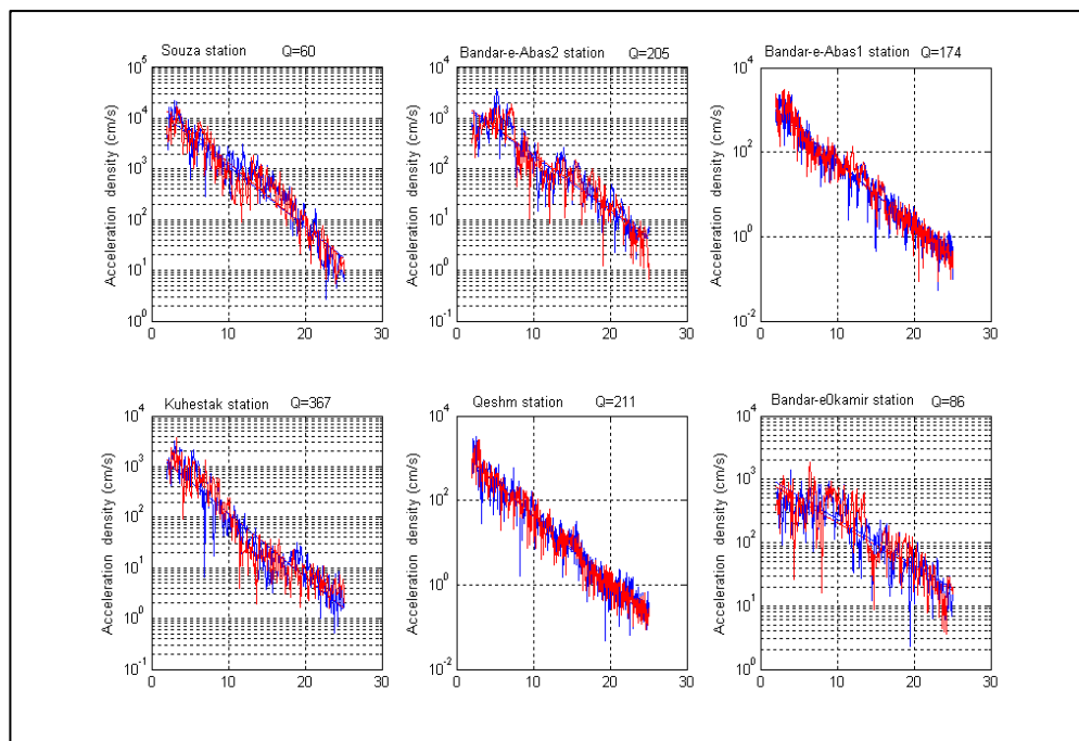
شکل ۴- برآورد عامل کیفیت برای مؤلفه‌های افقی ۶ ایستگاه زمین لرزه قشم (۲۰۰۵).
