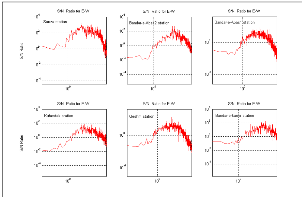
شکل ۳- برآورد نسبت سیگنال به نویز برای مؤلفه افقی رکوردهای زمین لرزه قشم (۲۰۰۵)
