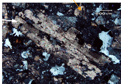
واحد تراکی آندزیتی دگرسان در نور پلاریزه
