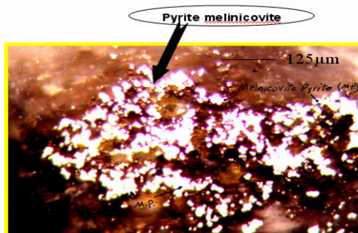
شکل ۹- تجمع دانه‌های کروی پیریت با منشأ ژله‌ای یا پیریت ملنیکوویت در نمونه شماره T4-6 با بزرگنمایی X250
