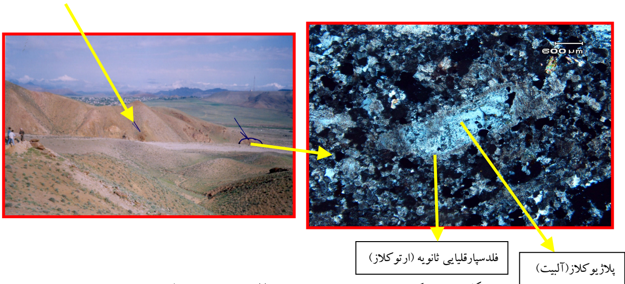
شکل ۳- واحد کوارتز مونزونیتی در محدوده مورد مطالعه دید به سمت شمال باختری
