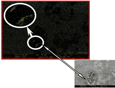
شکل ۱۵- پراکنندگی ذرات طلای ریز دانه در سطح مقطع و
