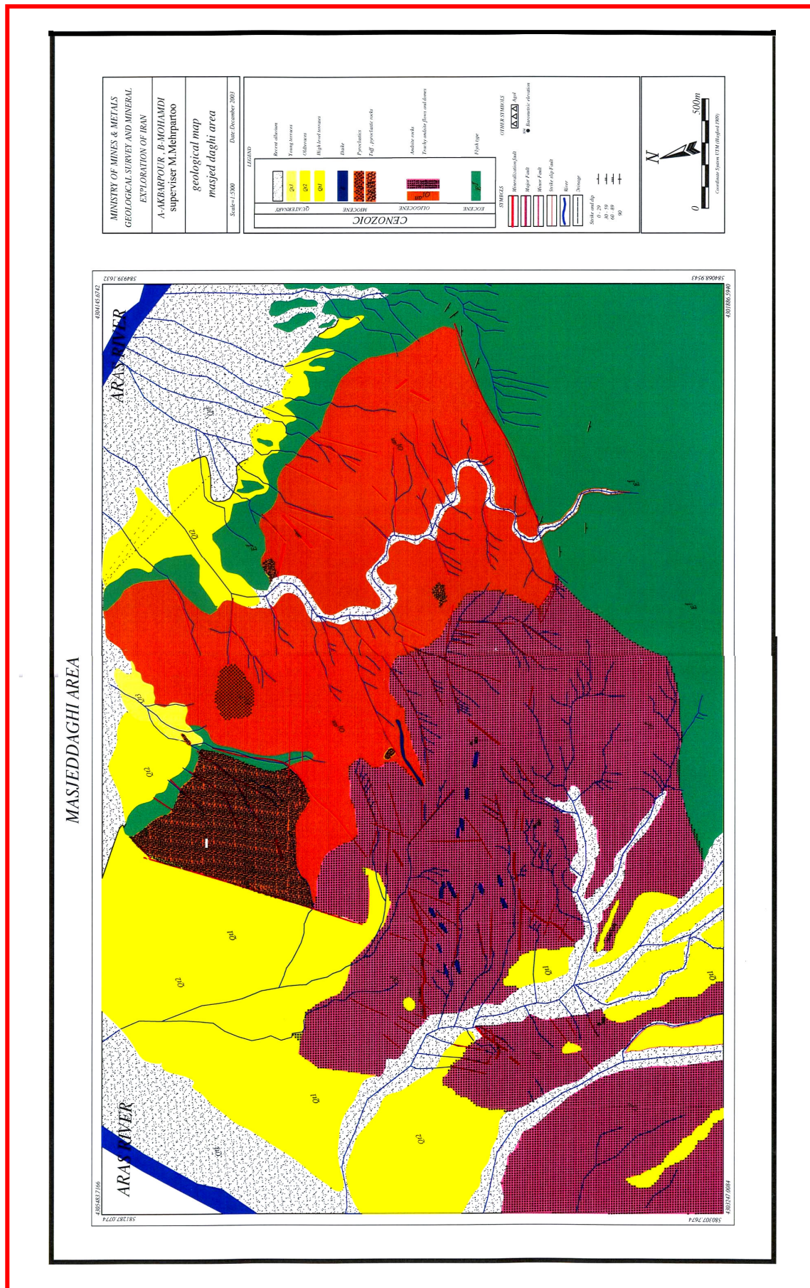
شکل ۱۸ - نقشه زمین شناسی با مقیاس ۱:۵۰,۰۰۰ محدوده مورد مطالعه
