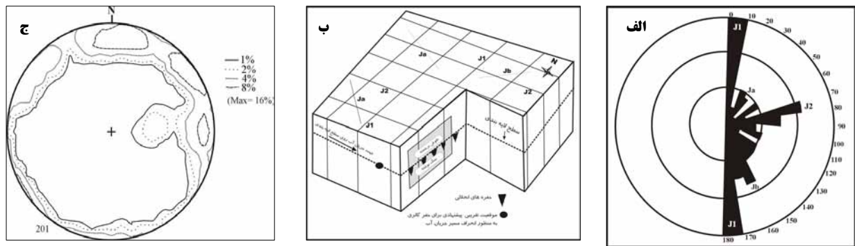
شکل ۴- الف) نمودار گلسرخی پراکندگی درزه‌ها در آهکهای پیرامون سنگ‌نوشته بیستون، ب) نمودار سه بعدی نشان دهنده موقعیت فضایی درزه‌های اصلی ( J_1, J_2 )، درزه‌های فرعی ( J_3, J_4 )، سطح لایه‌بندی با شیب به سوی سطح سنگ‌نوشته و موقعیت تقریبی حفره‌های انحلالی در حد فاصل نقش برجسته و سنگ‌نوشته. موقعیت پیشنهادی حفره‌گاری برای انحراف مسیر خروج آب از سطح سنگ‌نوشته در شکل مشخص شده است. ج) نمودار کنتوری درزه‌های منطقه پیرامون سنگ‌نوشته بیستون تا شعاع یک کیلومتری، برای جزئیات به متن مراجعه شود.
