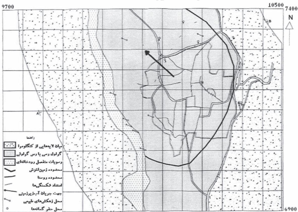
شکل ۲- نقشه زمین شناسی مهندسی زمین لغزش باریکان
