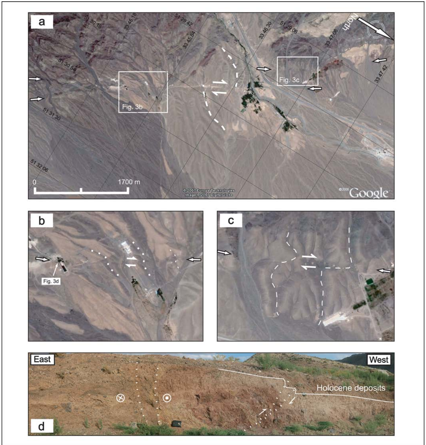
شکل ۳- (a) نگاره ماهواره‌ای (Google Earth) بخشی از قطع‌بندی گسلی کاشان در حوالی روستای گبرآباد. جهت پیکان‌ها راستای قطع‌بندی گسلی کاشان در این محدوده را بر روی نگاره نشان می‌دهد. به جابه‌جایی راست بر بادزن آبرفتی (در مرکز عکس) توجه کنید. (b و c) نمای نزدیک‌تر از خم شدگی و جابه‌جایی آبراهه‌ها در نتیجه عملکرد راست بر قطع‌بندی گسلی کاشان. (d) برش نهشته‌های بسیار جوان (کوآترنری و هولوسن) توسط شاخه‌های جوان قطع‌بندی گسلی کاشان در جنوب خاوری روستای گبرآباد. همان‌گونه که مشاهده می‌شود شیب گسل‌های رانندگی در این محل به سمت خاور است، یعنی خلاف جهت اصلی شیب گسل معکوس که به سمت باختر است.
