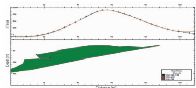
شکل ۶- مدل دو بعدی بی‌هنجاری D (RMS = 1/68) همراه با پاسخ مدل (منحنی سرخ رنگ) و داده‌های اندازه‌گیری شده (+ها)
