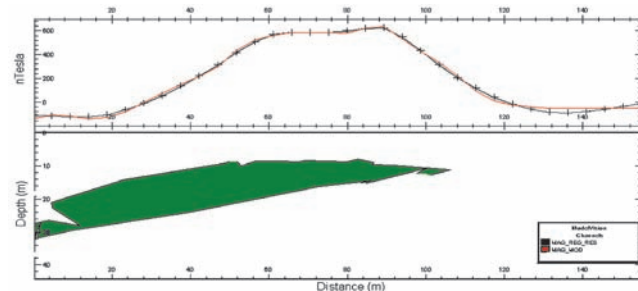
شکل ۵- مدل دو بعدی بی‌هنجاری A (RMS = 1/93) همراه با پاسخ مدل (منحنی سرخ رنگ) و داده‌های اندازه‌گیری شده (+ها)
