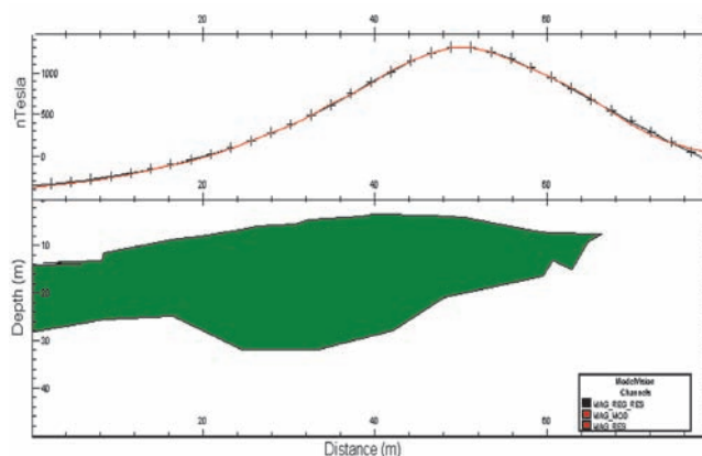
شکل ۷- مدل دو بعدی بی‌هنجاری F ( RMS = 1/391 ) همراه با پاسخ مدل (منحنی سرخ رنگ) و داده‌های اندازه‌گیری شده (+ ها)
