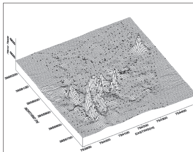
شکل ۳- نمایش سه بعدی میدان کل مغناطیسی همراه با محل برداشت داده‌ها (نقاط مشکلی) و نمونه‌ها (نقاط آبی)
