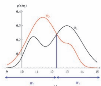
شکل ۲- افزایش فضای تصمیم بر اساس احتمال شرطی، الف) در حالتی که توزیع احتمال شرطی گوسی است (Duda et al., 2003) ب) در حالتی که توزیع
