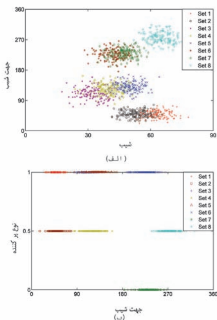
شکل ۸- نمودارهای دوبعدی تمرکز ویژگی های دسته درزه های ۸ گانه بر اساس دو ویژگی (الف) شیب و جهت شیب، (ب) جهت شیب و نوع پرکننده.
