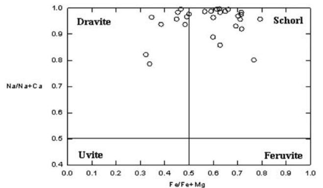
شکل ۷- نسبت Na / (Na + Ca) در برابر Fe/ (Fe + Mg) (Hawthorne & Henry, 1999) نمونه‌های مورد مطالعه در محدوده شورلیت و دراویت و با تمایل بیشتر به سمت شورلیت قرار می‌گیرند.
