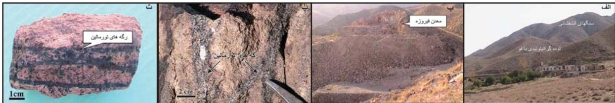
شکل ۲- الف) نمای دور از روستا و توده گرانیتویدی باغو، دید به سمت جنوب خاور، ب) معدن فیروزه در توده داستیتی، دید به سمت جنوب، پ) رگه‌های کوارتز- تورمالین در توده گرانیتی باغو و ت) رگه‌های غنی از تورمالین در نمونه دستی.
