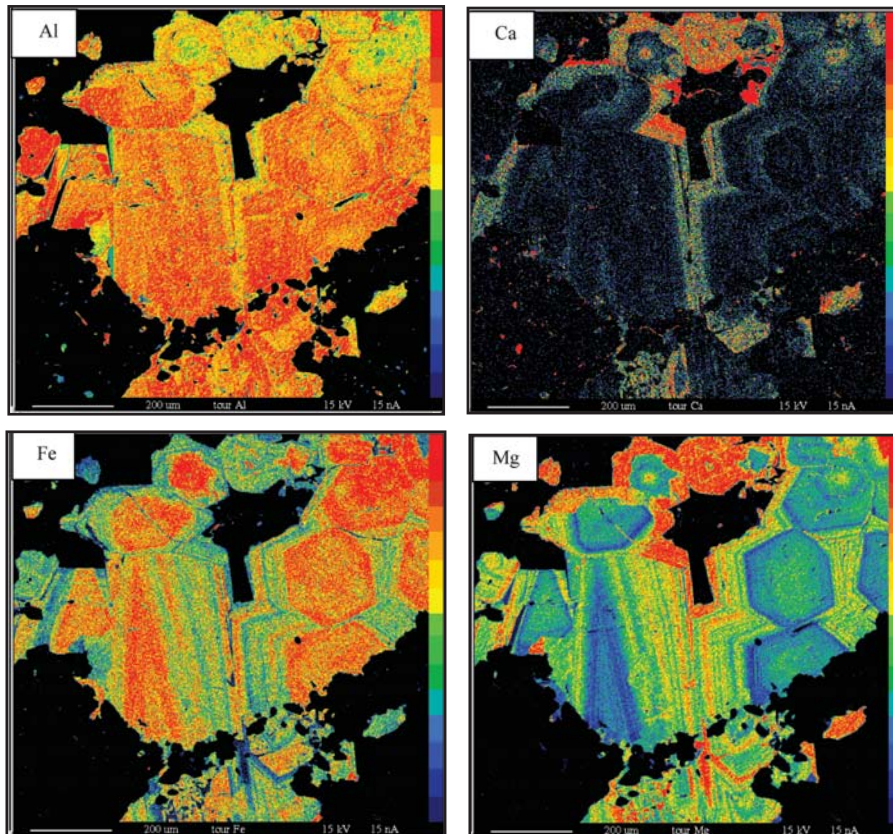
شکل ۱۲ - نقشه‌های اشعه ایکس توزیع عناصر Mg، Al، Ca و Fe، در تورمالین‌های مورد مطالعه که نشان‌دهنده آن است که بلورهای تورمالین دارای زون‌بندی متحدالمرکز هستند. نقشه‌ها با استفاده از ولتاژ شتاب‌دهنده 15 kV و جریان پرتو 15 nA به دست آمده است. شمارش در هر ثانیه برای هر عنصر اندازه‌گیری شده و در حاشیه سمت راست نقشه با استفاده از مقیاس رنگ، از سیاه تا قرمز به ترتیب برای شمارش‌های کم تا زیاد پلات شده است.
