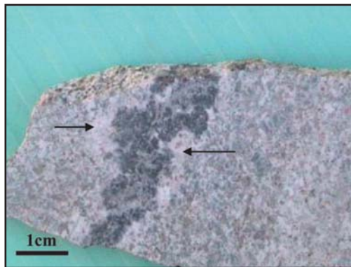
شکل ۴- وجود بخش هاله روشن در همبری سنگ گرانیتی و تورمالین در نمونه دستی که با فلش نمایش داده شده است.
