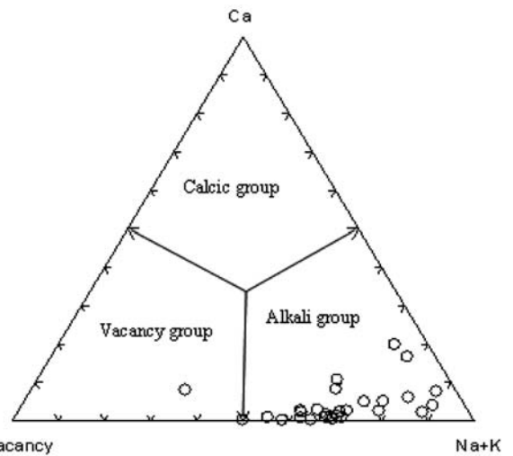
شکل ۵- ترکیب تورمالین‌های مورد مطالعه در نمودار مثلثی Ca ، Na + (K) و X-Site vacancy (Hawthorne & Henry, 1999). بیشتر نمونه‌های مورد مطالعه در قلمرو تورمالین‌های قلیایی قرار می‌گیرند و فقط یک نمونه در قلمرو گروه Vacancy واقع شده است. (X_{vac} (X_{vacancy}) = 1 - (Na + K + Ca)) .
