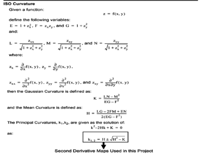
شکل ۶- محاسبات ریاضی به کار رفته در نقشه‌های حاصل از روش نشانگر مشتق اول و دوم جهت دار افقی‌های تفسیر شده.
