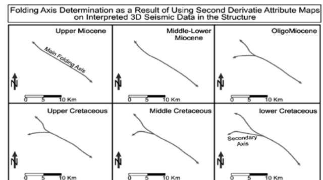
شکل ۷- نتایج نقشه مشتق دوم بر افقی‌های تفسیر شده در ساختمان مورد نظر. به پیدایش پلانژ سوم در افق الیگومیوسن و گسترش آن به سمت افقی‌های پایین‌تر که با خمیدگی ناگهانی به سمت جنوب باختر همراه است، دقت کنید.
