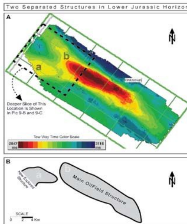
شکل ۷- مشاهده مستقیم ساختار تداخلی پوشیده شده به وسیله ساختمان اصلی در بخش جنوبی دماغه شمال باختری، بدون استفاده از نشانگرهای لرزه‌ای در ژرف‌ترین افق تفسیر شده.
