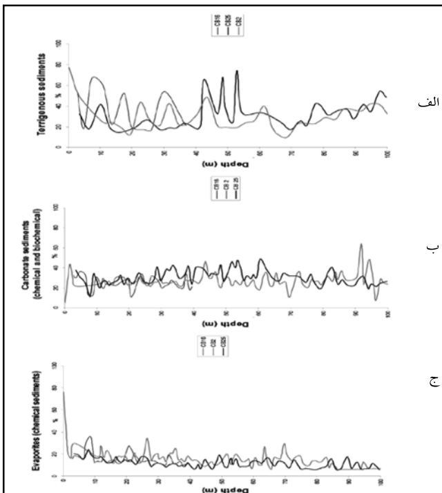
شکل ۶- پراکندگی ذرات آواری (الف)، کربناته (ب) و تبخیری (ج) در مغزه‌های مورد مطالعه و تغییرات فراوانی آنها در طول گمانه‌ها. مقادیر ارائه شده برای هر ذره میانگین به دست آمده از چهار گمانه است.
