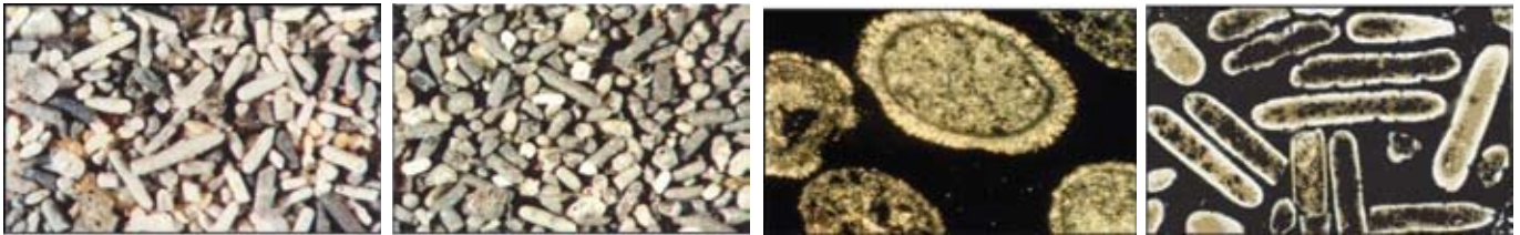
شکل ۴- نمونه‌ای از پلت‌های مدفوعی (fecal pellets) موجود در مغزه‌های مورد مطالعه. الف) پلت‌های میله‌ای (شکسته و سالم) با ترکیب آراگونیتی مربوط به لایه‌های بالایی مغزه‌ها که به طور بخشی در سطح دچار خوردگی شده‌اند (تصویر استریومیکروسکوپ، بزرگنمایی ۳۰). ب) تصویر میکروسکوپی از پلت‌های موجود در لایه‌های زیرین مغزه‌ها که ترکیب آراگونیتی با ماهیت شعاعی به خوبی در آن مشخص است. بخش‌های تیره در مرکز، افق‌های پیریتی شده را نشان می‌دهند (نور پلاریزه، بزرگنمایی ۴۰).
