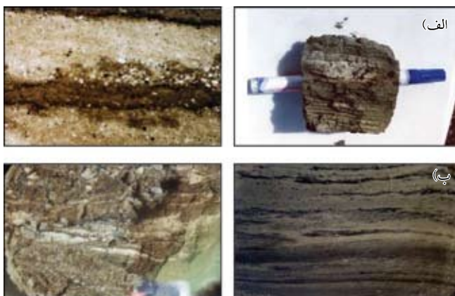
شکل ۹- الف) ذرات آواری موجود در نمونه‌های مورد مطالعه که به طور عمده دارای شکل بلوری منظم تا نیمه منظم هستند (تصویر استریو میکروسکوپ با بزرگنمایی ۳۰). تصویر SEM از ذرات آواری حاوی بلورهای اتومورف پیروکسن (ب) و کوارتز (ج).
