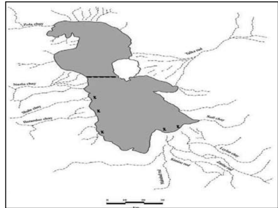
شکل ۲- موقعیت رودخانه‌های اصلی تغذیه کننده دریاچه نسبت به محل میانگذر و محل‌های نمونه‌برداری در دهانه رودخانه‌ها
