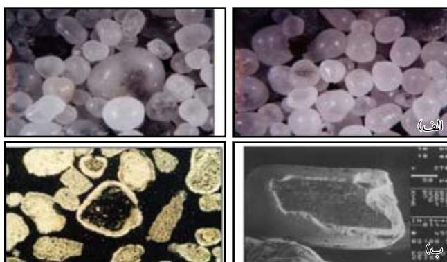
شکل ۸- الف) ذرات پوشش دار ژیس با شکل کروی در حد گراول (ذرات شیمیایی) با هسته‌ای از ذرات آواری (چپ) و فاقد هسته (راست). ب) تصویر میکروسکوپی از ذرات پوشش دار با گسترش قشر آراگونیتی در اطراف شیشه آتشفشانی (چپ)، و تصویر SEM از گسترش قشر کربناته در اطراف یک قطعه آواری فلدسپار (راست).
