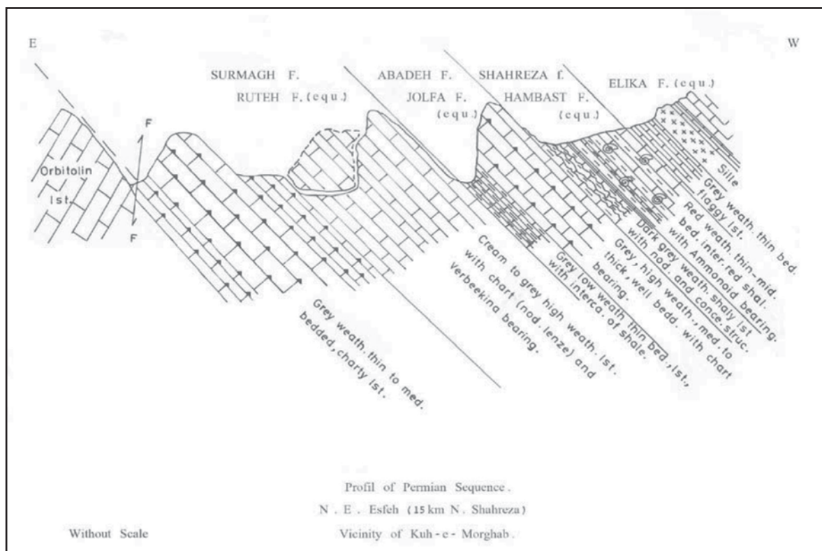
شکل ۳- مقطع عرضی برش اسفه www.SID.ir
