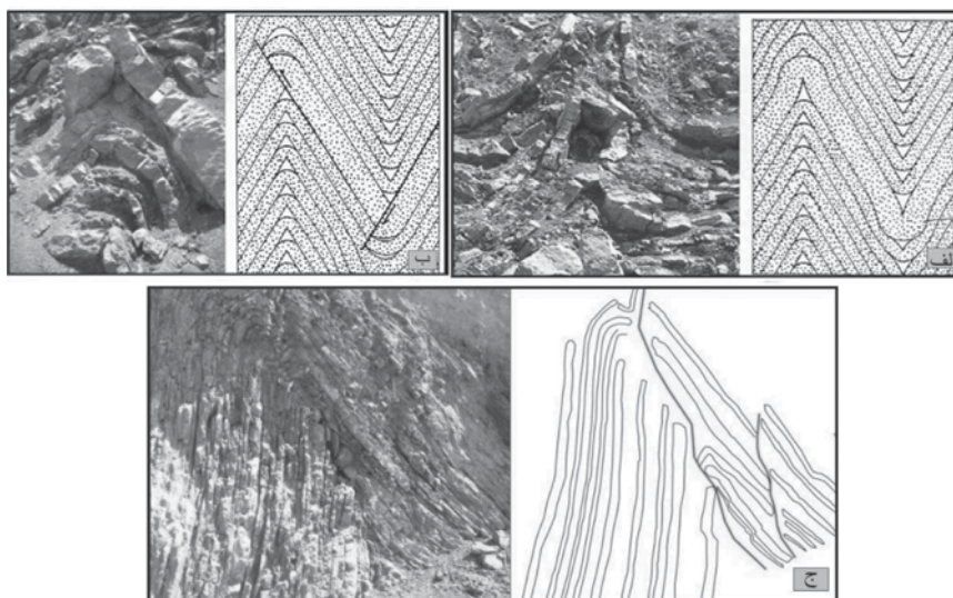
شکل ۶- الف) bulbo hinge structure (ب) limb thrust (اشکال سمت راست در الف و ب با اقتباس از Ramsay & Huber, 1987) در بخش میانی حوضه رادیولاریتی، نگاه به سمت خاور. ج) ساختار limb thrust در چین‌های جناغی پهنای شکل حدود هفت متر، نگاه به سمت جنوب خاوری. در بخش میانی حوضه رادیولاریتی، نگاه به سمت خاور.
