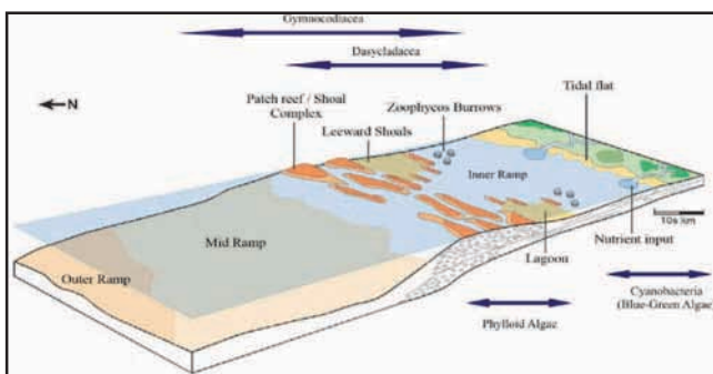
شکل ۵- پراکنندگی جلدک‌های آهکی در نیمرخ رمپ کرنباتی هم‌شیب، پرمین البرز مرکزی
