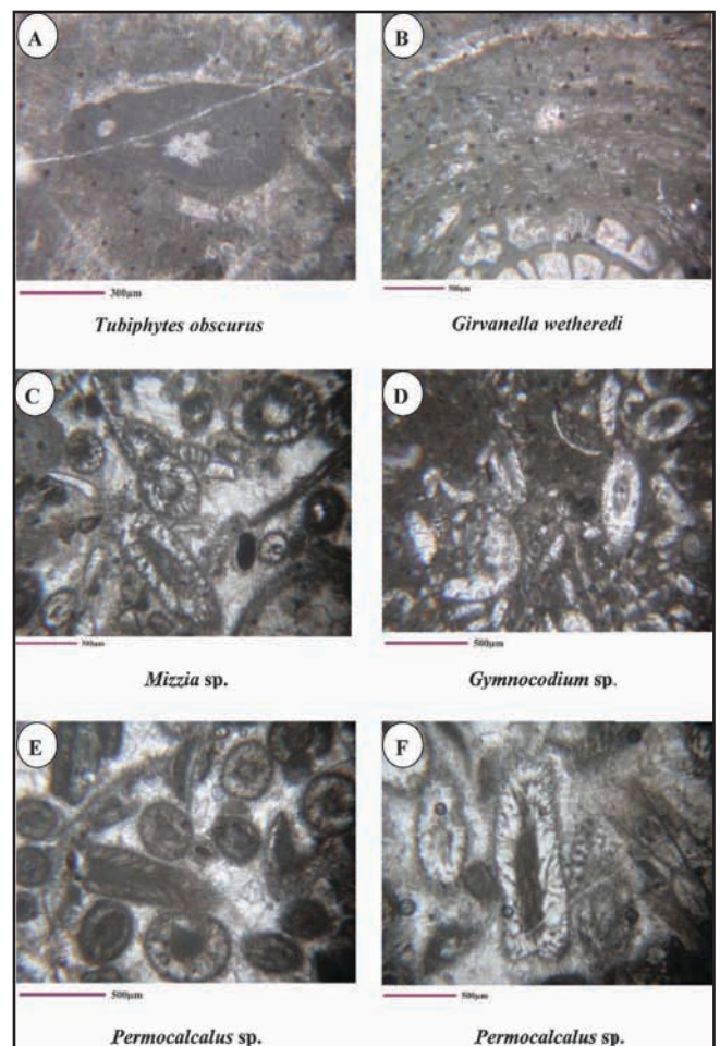
شکل ۳- جلدک‌های آهکی پرمین در برش گدوک البرز مرکزی
