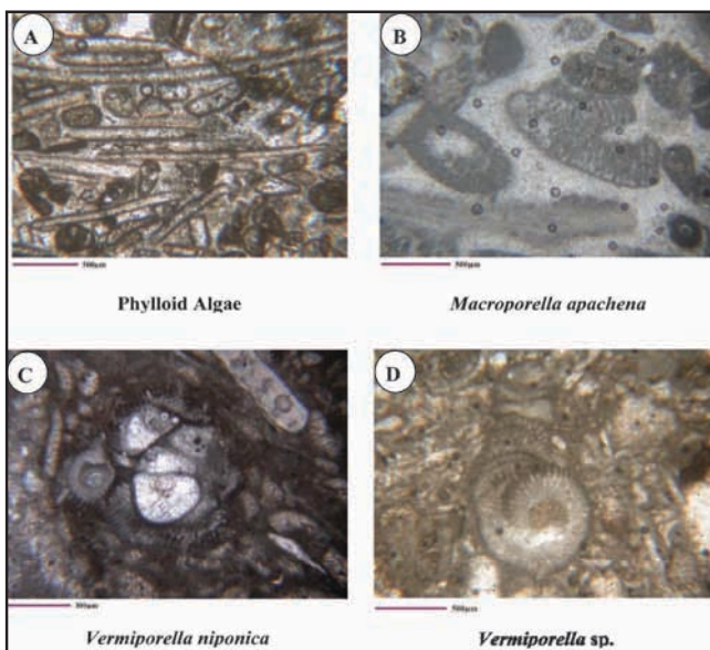
شکل ۴- جلدک‌های آهکی پرمین در برش گدوک البرز مرکزی
