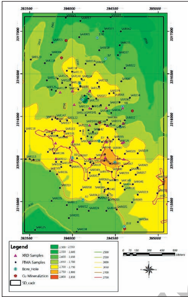
شکل ۳- مدل ارتفاع رقومی و منحنی های میزان توپوگرافی همراه با موقعیت منطقه نمونه برداری PIMA-ICP و XRD.
